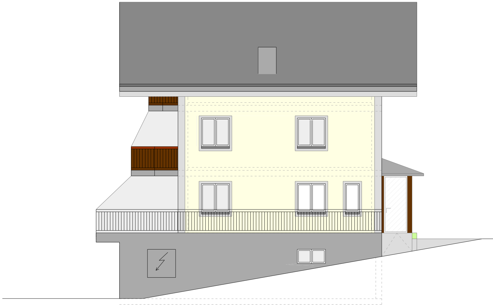
OST-FASSADE 1:100
